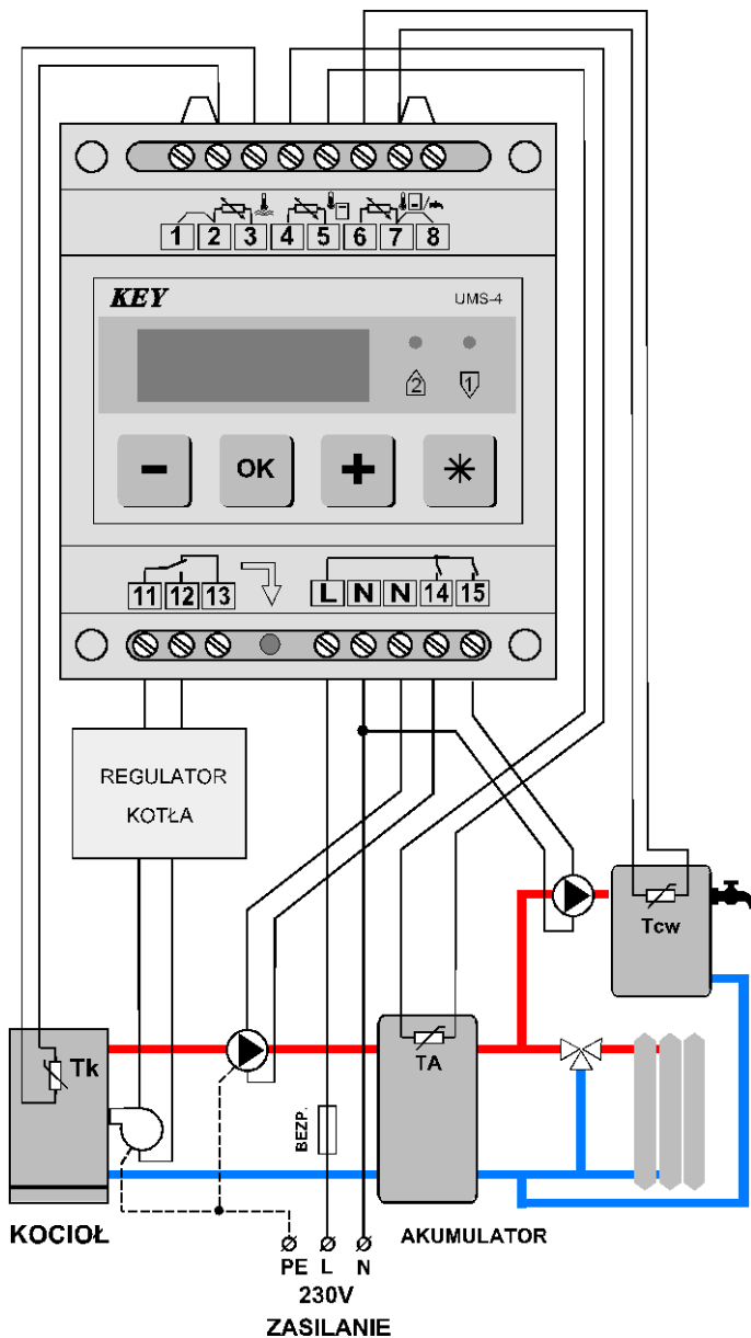
Rysunek 3. Schemat podłączenia modułów UMS-4A w układzie zawierającym zasobnik CWU zasilany z akumulatora.
