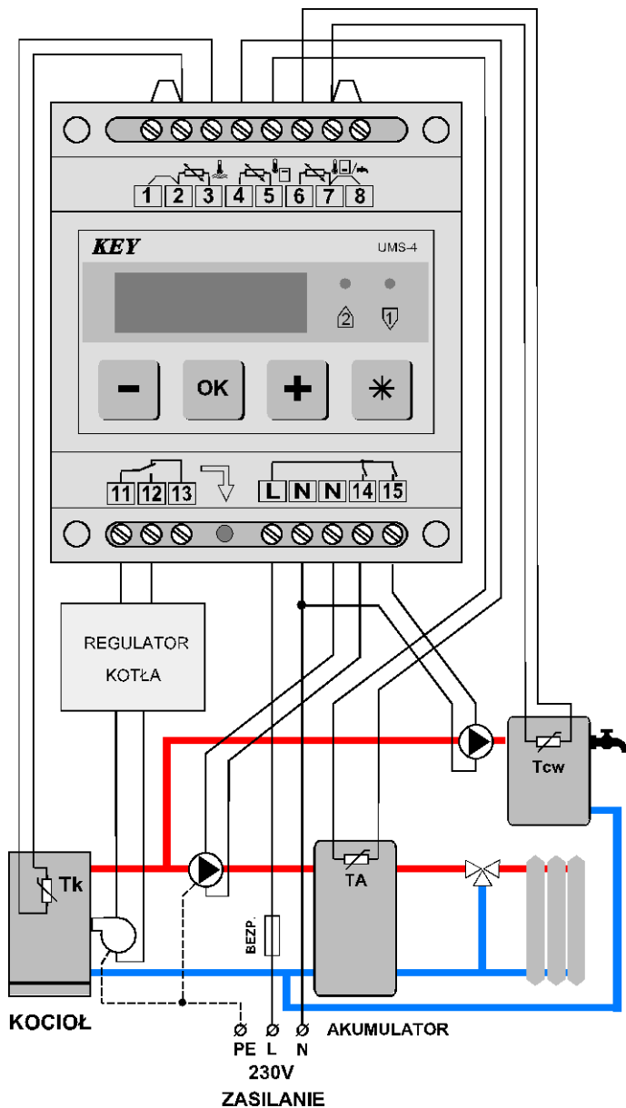
Rysunek 4. Schemat podłączenia modułów UMS-4A w układzie zawierającym zasobnik CWU zasilany z kotła.
