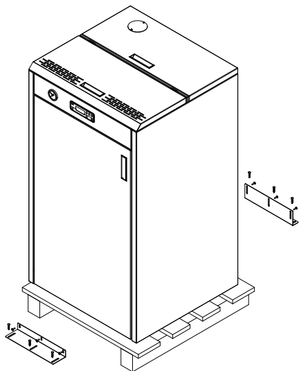
RYSUNEK 1 - WYJIMOWANIE ŚRUB Z OPAKOWANIA
