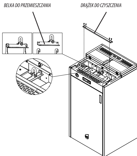
RYSUNEK 2 - ZACZEP DO PRZEMIESZCZANIA
