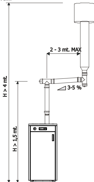
PRZYKŁAD INSTALACJI KOTŁA NA PELETY
